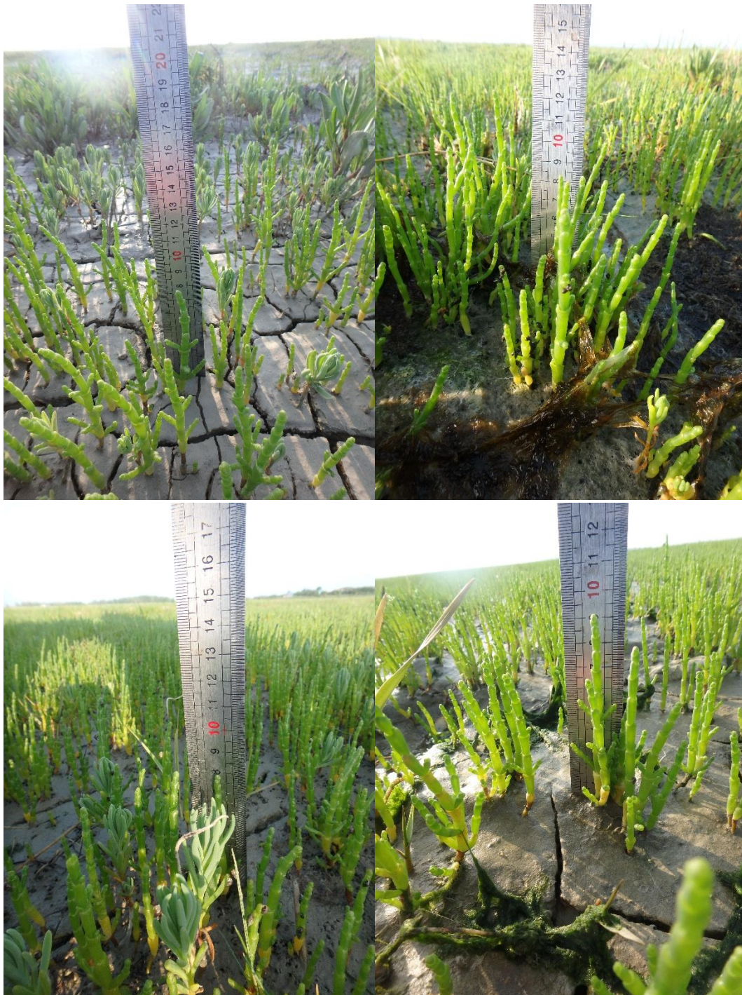
Figure 1 : Photos de salicornes observées dans la zone travaillée du Hourdel
